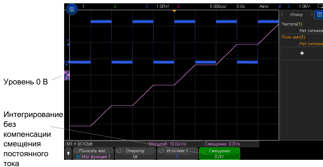
Рис. 9 Интегрирование без смещения сигнала
